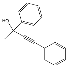
2,4-DIPHENYL-3-BUTYN-2-OL
