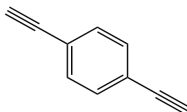
P-DIETHYNYLBENZENE
